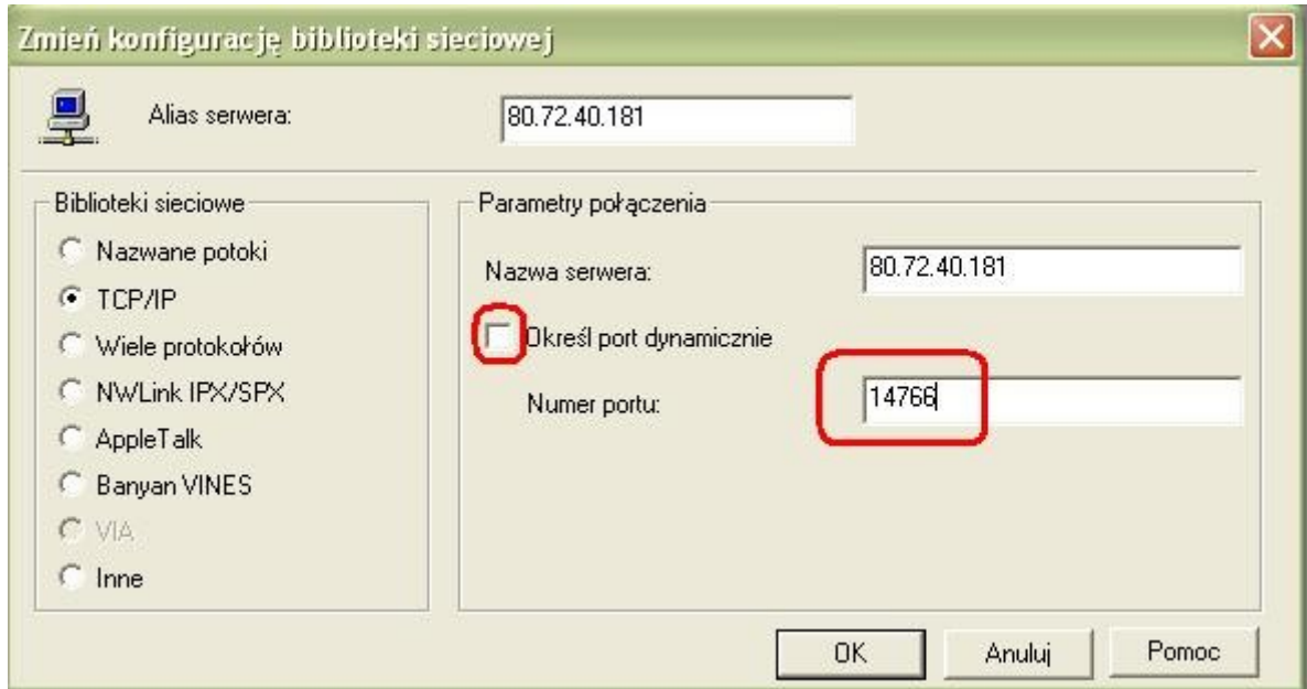
Rysunek 5. Konfiguracja klienta
